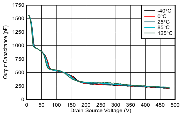
图 5-8. 输出电容与漏源电压之间的关系
