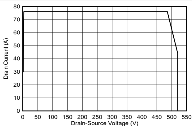
图 5-11. 最大安全工作区
