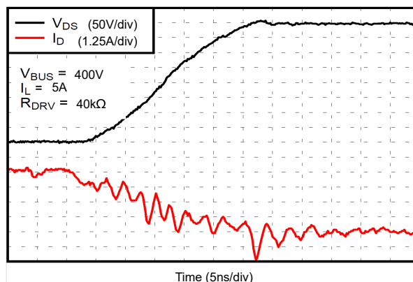
图 8-6. 应用示例中的关断波形
