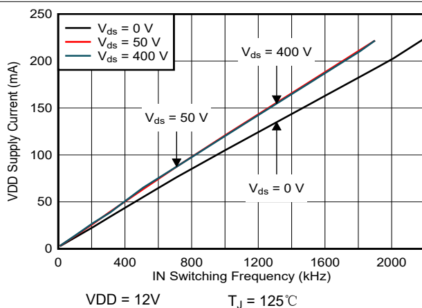
图 5-10. VDD 电源电流与输入开关频率之间的关系
